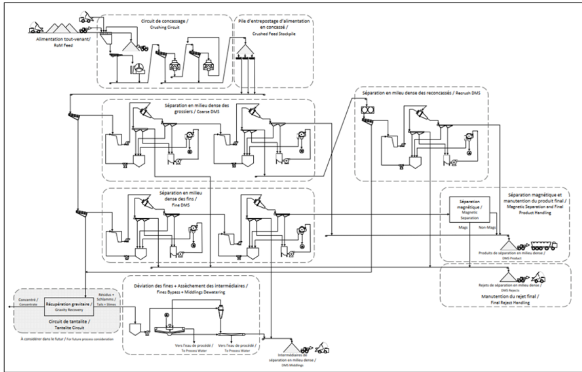
Figure 1 Diagramme de procédé de traitement simplifié
